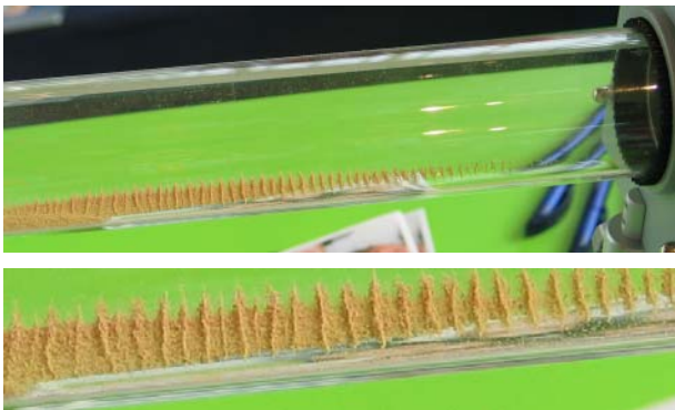
Abb. 08: Korkmehl und stehende Wellen in einem akustischen Rohr, Anregung über einen Lautsprecher rechts. Das Mehl bleibt dort liegen, wo die Luftteilchen kaum in Bewegung sind. Es bilden sich scharfkantige Haufen. Schaltet man die Anregung ab und klopft auf das Rohr, fallen die Haufen zusammen, das Mehl verteilt sich wieder.
