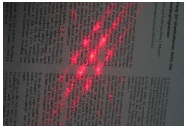
Abb. 02: Laserstrahl durchleuchtet ein dünnes Seidentuch. Es entsteht in einigen Metern Entfernung ein gut sichtbares, komplexes Beugungsbild (Interferenzbild). Die Anordnung der Punkte und deren Lichtverteilung erlaubt eine Aussage über die Geometrie der Maschen und Fäden des Tuches sowie zur Symmetrie des Gewebes. Eine graphische Manipulation der Position eines Punktes würde man sofort als Fehler entlarven können, wenn dadurch die Symmetrie verletzt wird.
