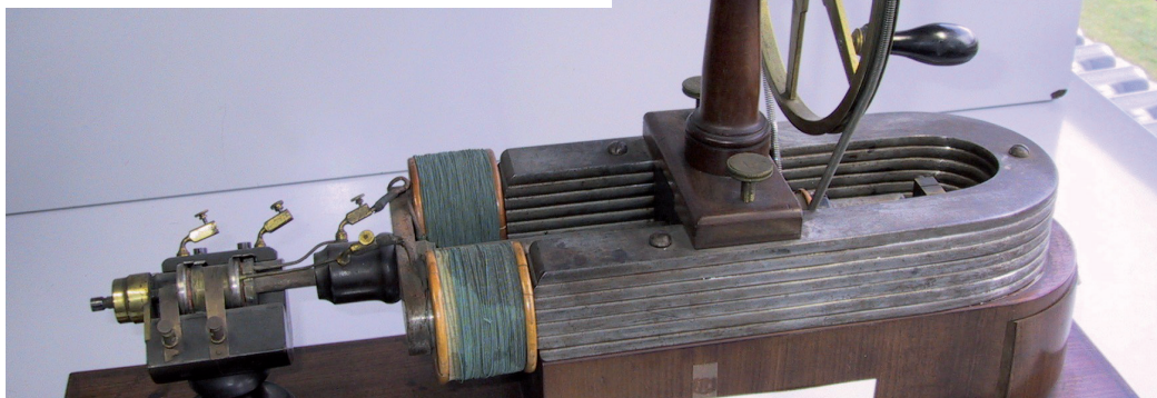
Abb. 08: Induktionsapparat (Wechselstromgenerator) aus dem 19. Jahrhundert, gebaut u.a. für medizinische Zwecke der Fa. Dr. Störcher Leipzig. Der Hufeisenmagnet besteht aus sieben Lagen geschmiedeten Eisens. /Balck 2011/
