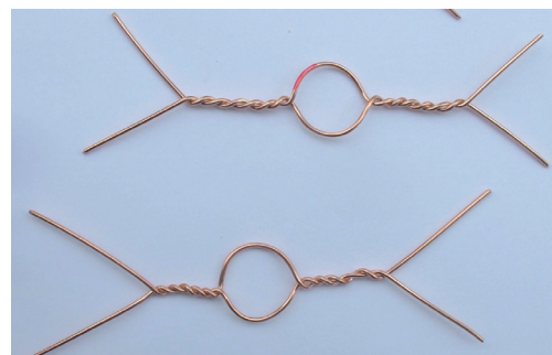
Abb. 18: andere Bauform, Nachbau aus Kupferdraht, unterschiedliche Drehrichtung der Verdrillung /Korschelt 1892/ S. 167
