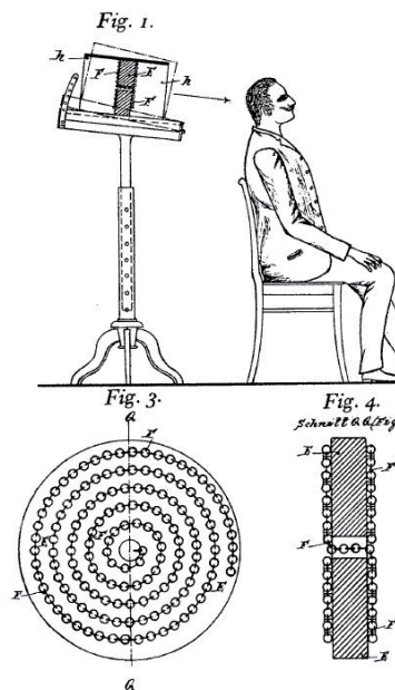
Abb. 16: Ätherstrahlapparat von Korschelt, Patent DRP 69340.
